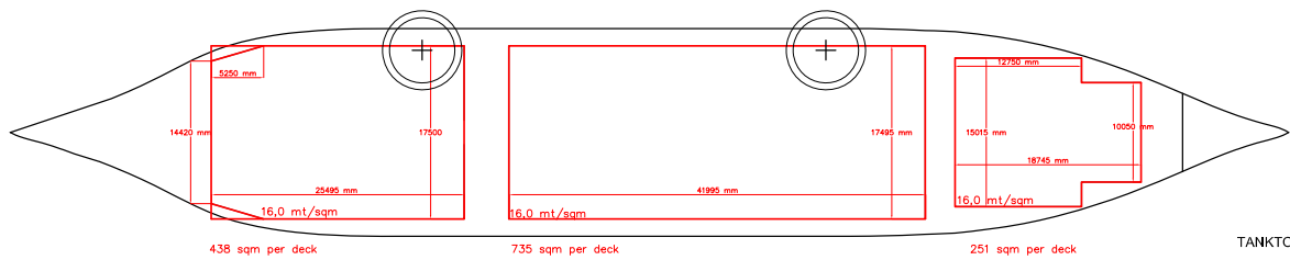
TWEENDECK
